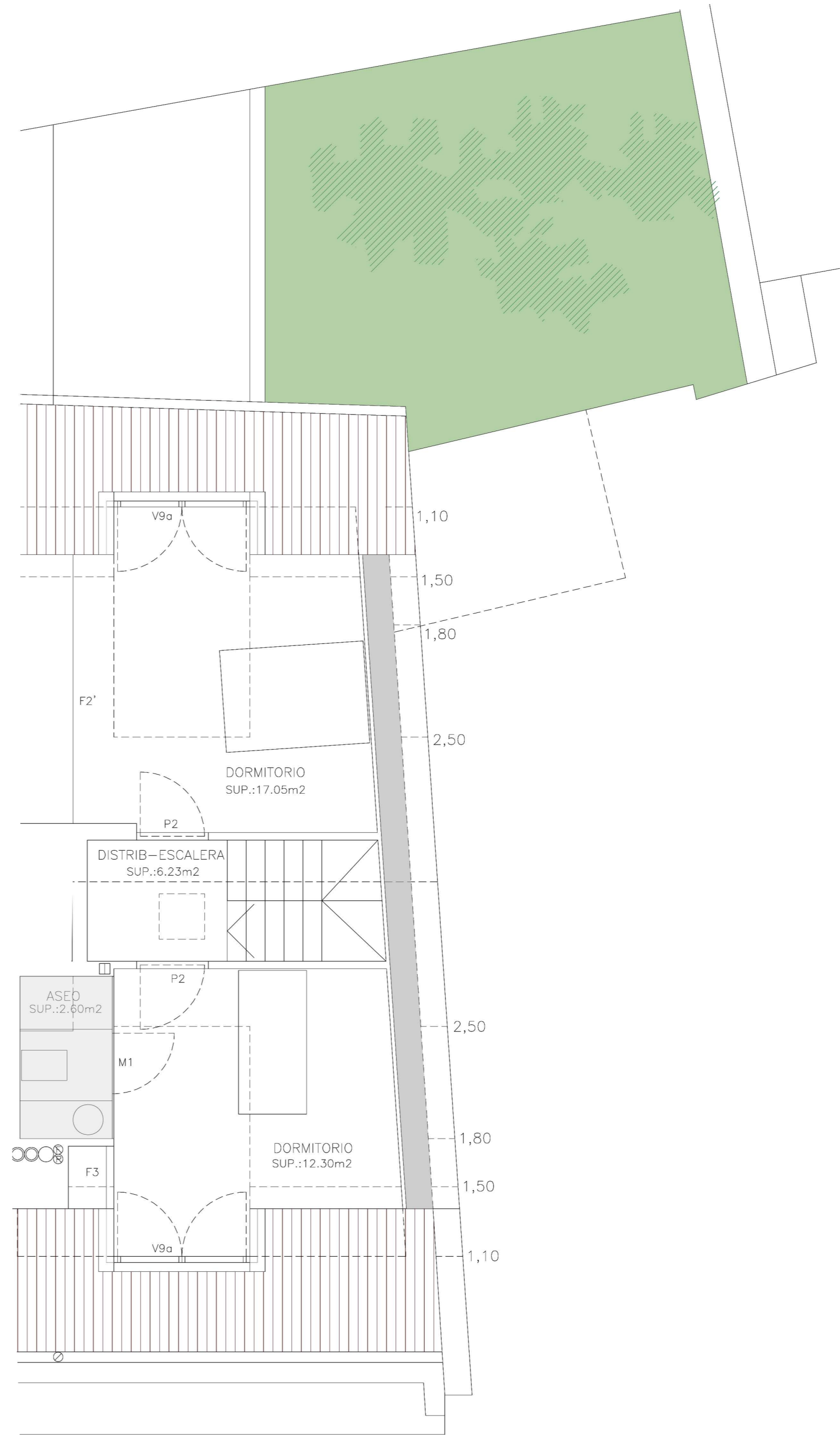
BAJO CUBIERTA
