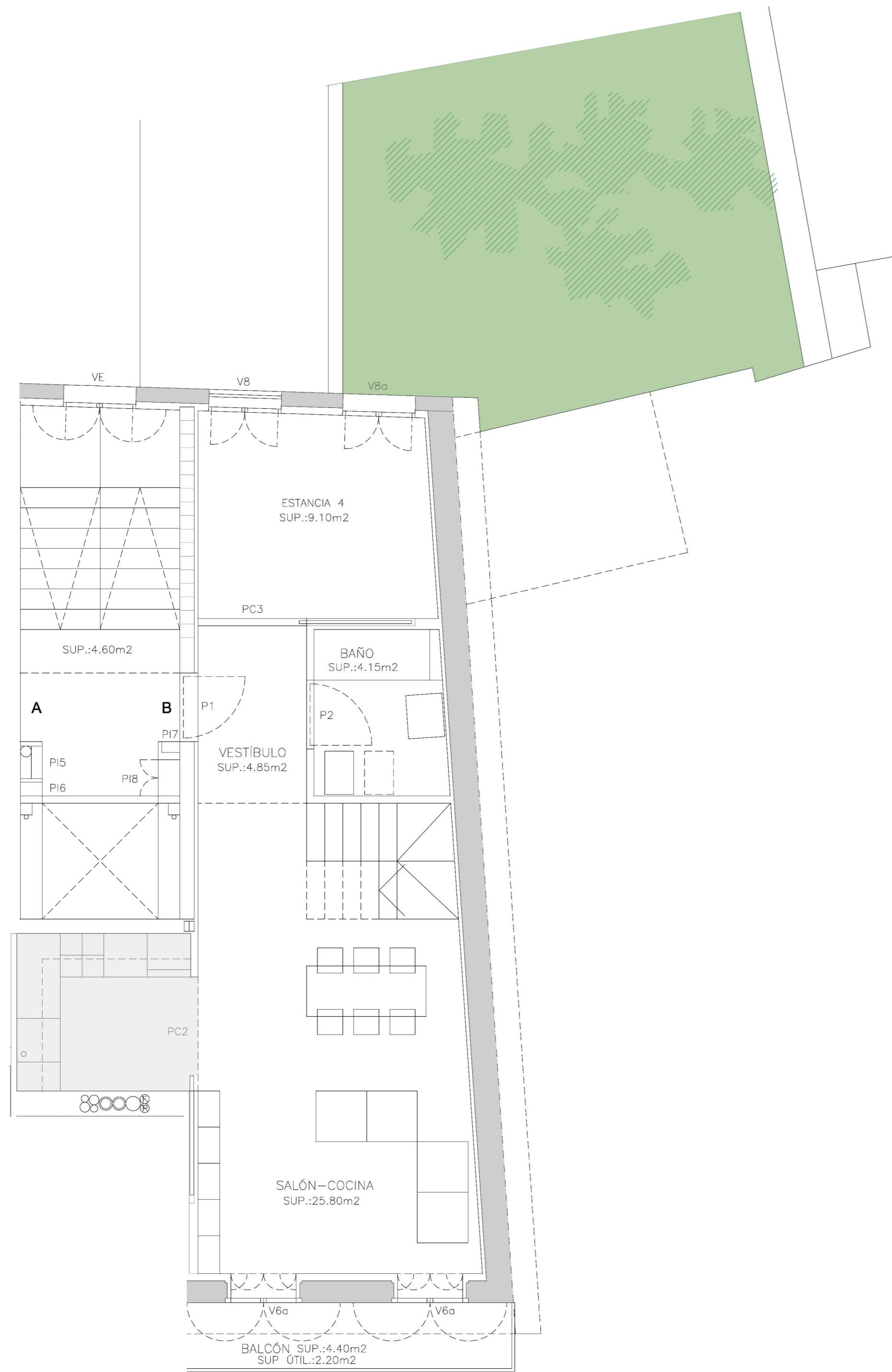
PLANTA SEGUNDA
