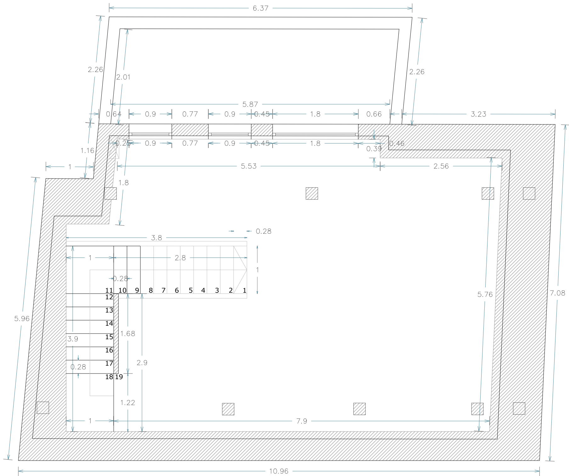
PLANTA SEMISÓTANO E: 1/50
