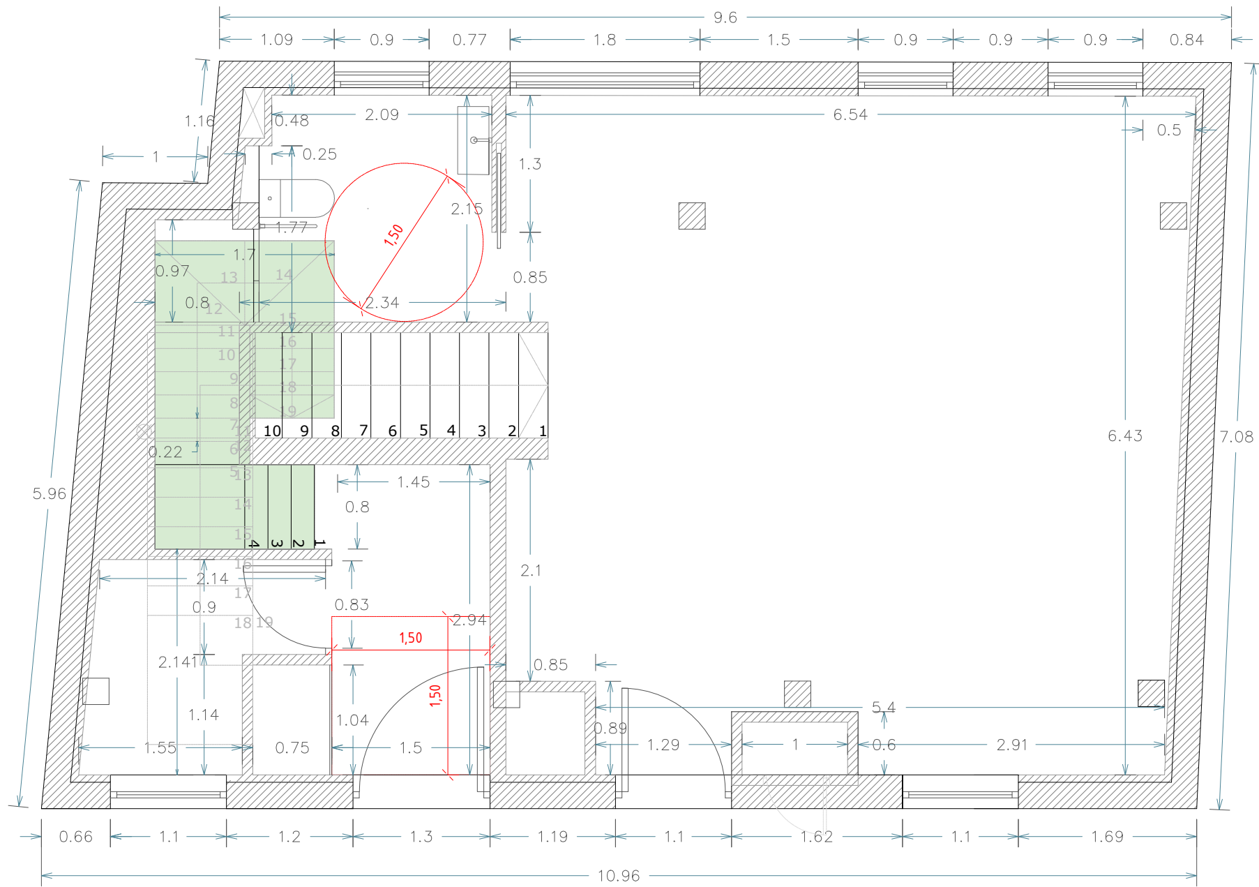
PLANTA BAJA E: 1/50
