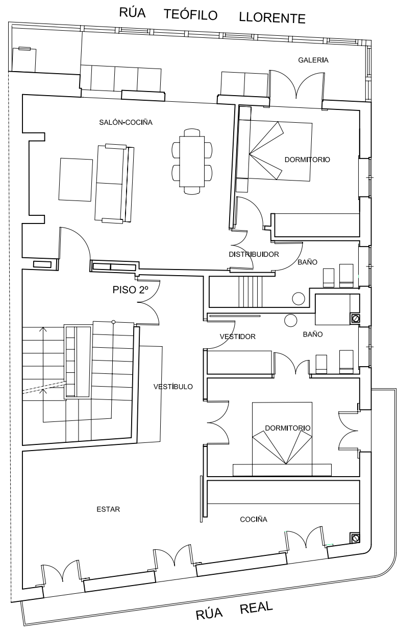
SEGUNDO ANDAR ESCALA 1/100
